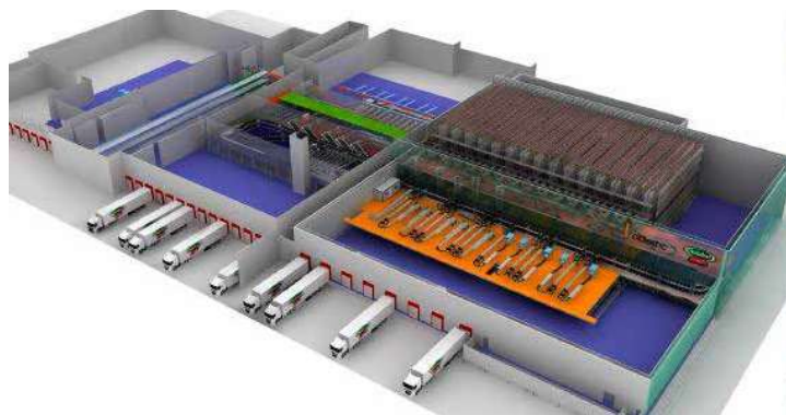
Il rendering del nuovo polo logistico di Amadori
